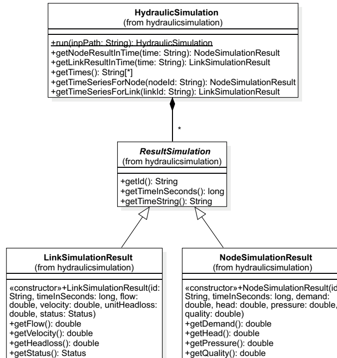
Figura 4.6: Diagrama de clases para la simulación hidráulica
