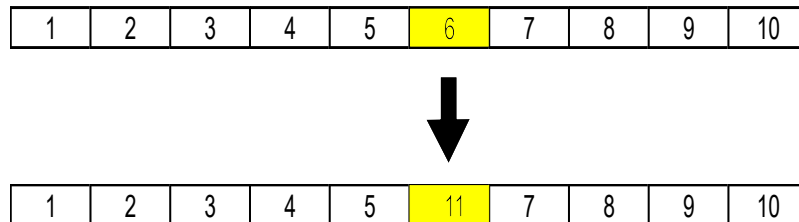
Figura 2.7: Mutación aleatoria
