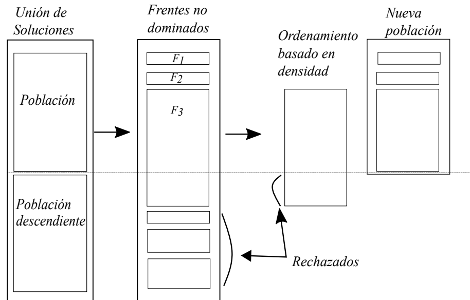
Figura 2.10: Procedimiento NSGAI [34]
