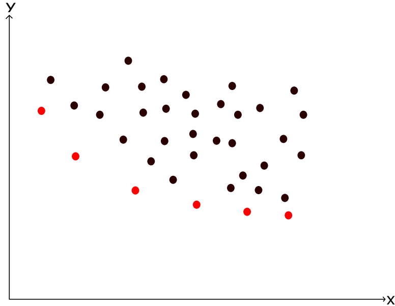
Figura 2.5: Ejemplo frente de Pareto
