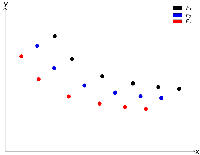
Figura 2.11: Frentes no dominados
