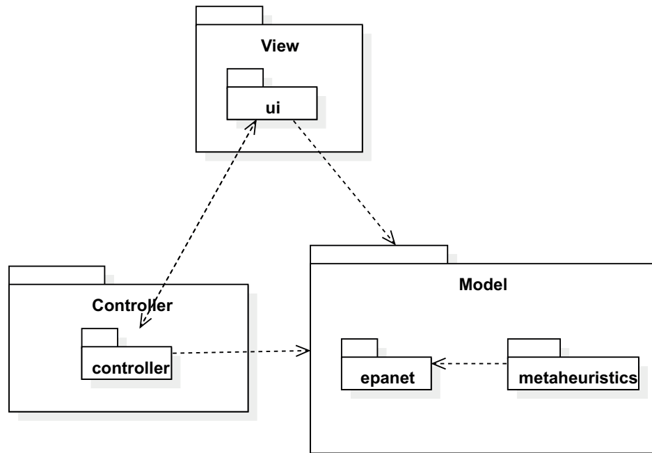
Figura 4.2: Arquitectura lógica Modelo-Vista-Controlador
