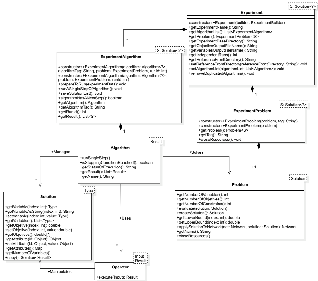
Figura 4.4: Diagrama de clases modulo metaheurística. Modificación a partir del diagrama presentado en [4]
