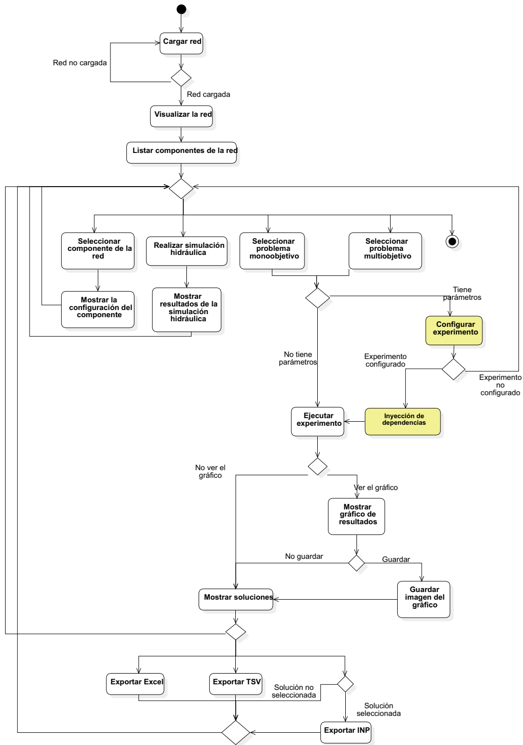
Figura 4.8: Diagrama de actividades de la aplicación
