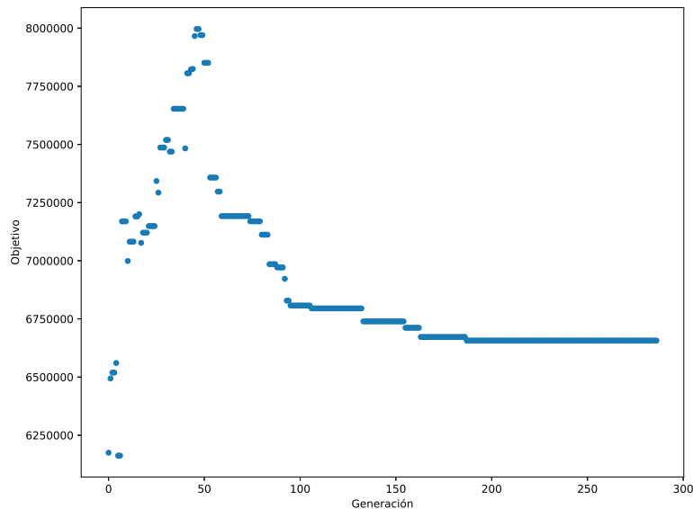
Figura 2.3: Gráfica objetivo versus generación para un problema
