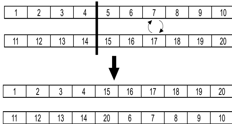
Figura 2.6: Cruzamiento en un punto
