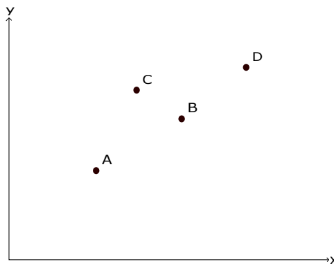
Figura 2.4: Ejemplo de dominancia y Óptimo de Pareto
