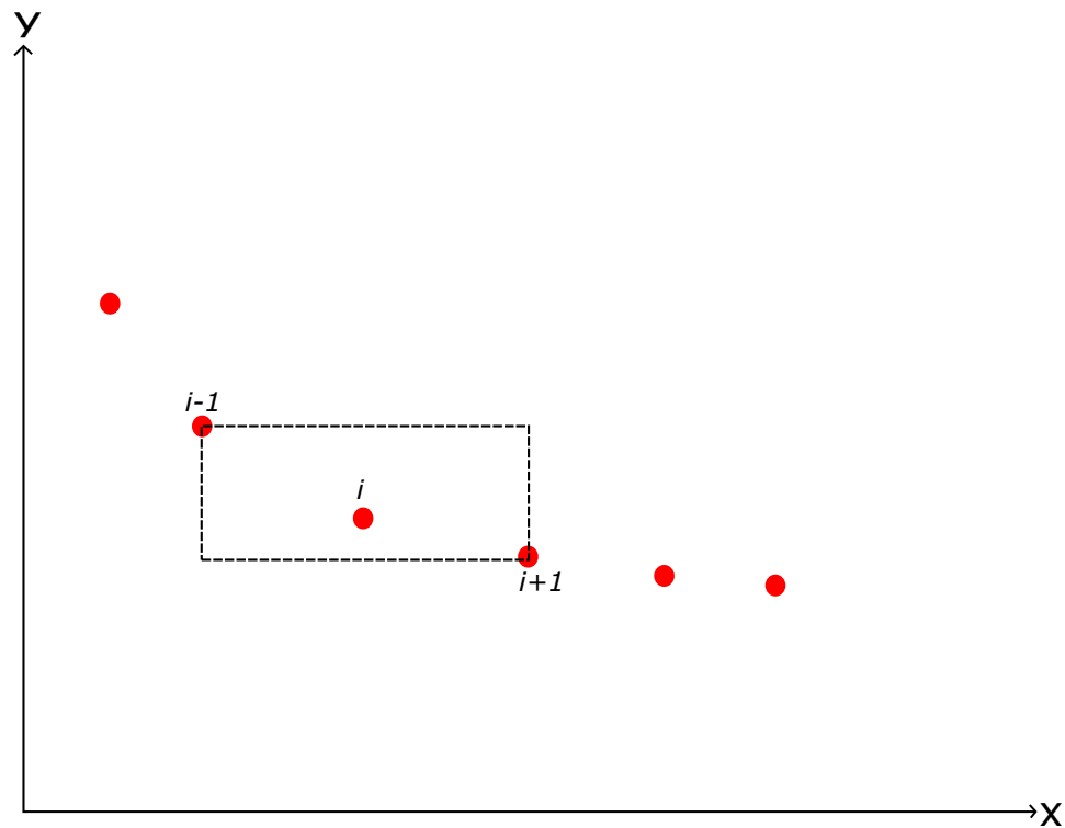
Figura 2.13: Cálculo de la densidad de estimación al rededor de la solución i [34]
