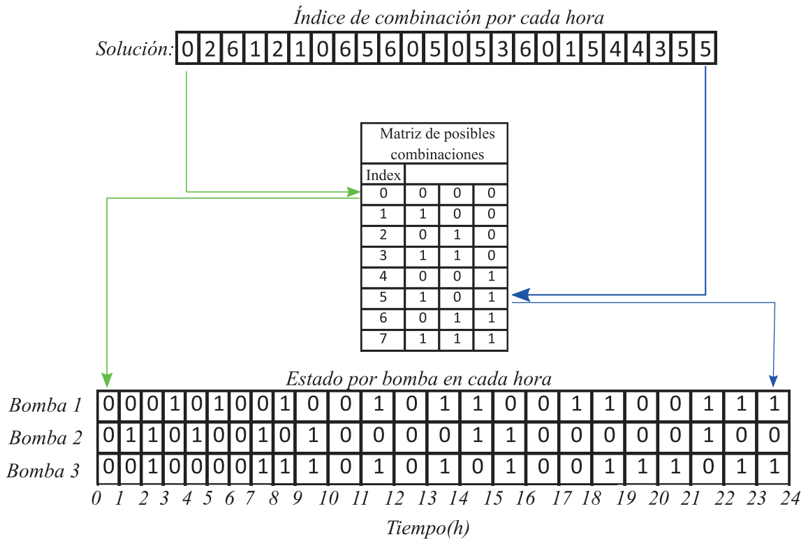
Figura 2.16: Representación de la solución problema multiobjetivo Pumping Schedule
